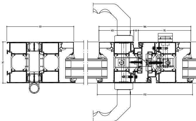
Sezione orizzontale
